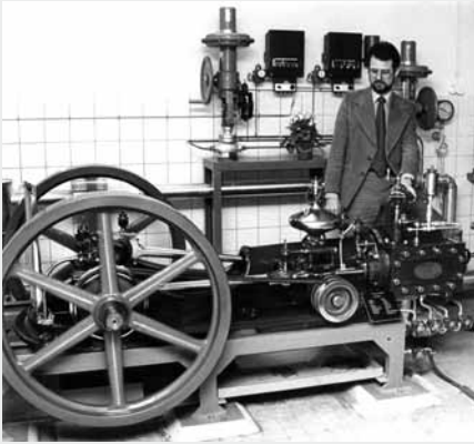
SIEGBERT SEMLING, TS-DIPLOMAND, MIT DER RESTAURIERTEN DAMPFMASCHINE.
